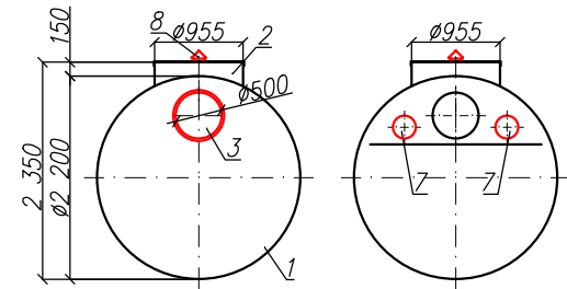
Вид спереди
